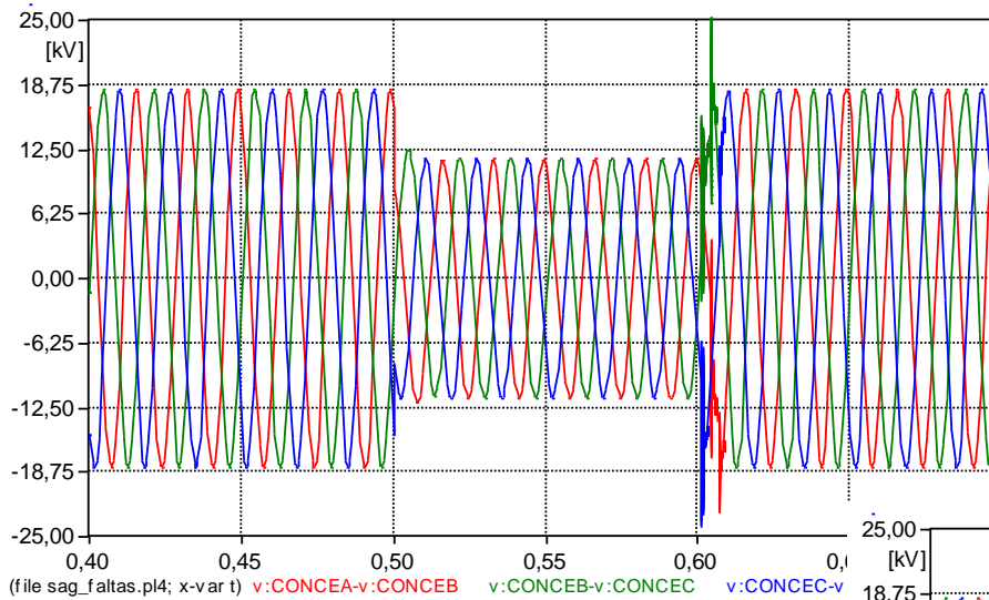
Falta trifásica
